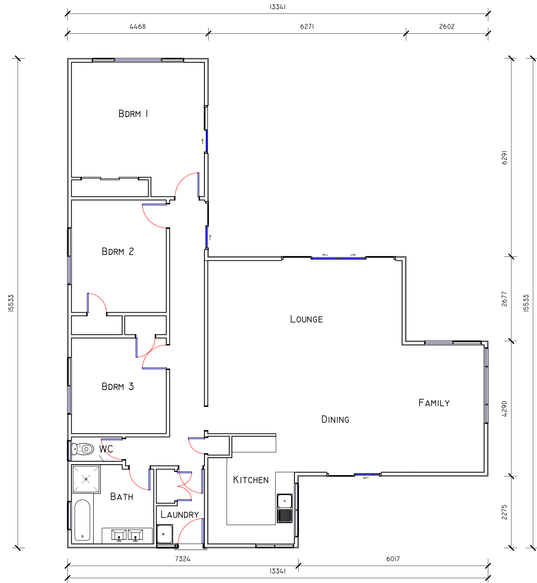
① Layout 1 : 75
